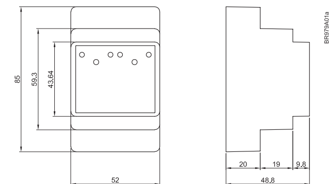
Abmessungen (mm)
